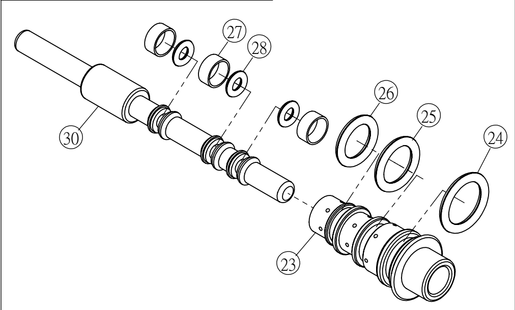
23-30|BodyOfThimbleValve Set|1|A31-23N30N
